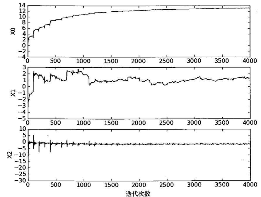
图5-7 使用样本随机选择和alpha动态减少机制的随机梯度上升算法stocGradAscent1()所生成的系数收敛示意图。该方法比采用固定alpha的方法收敛速度更快
