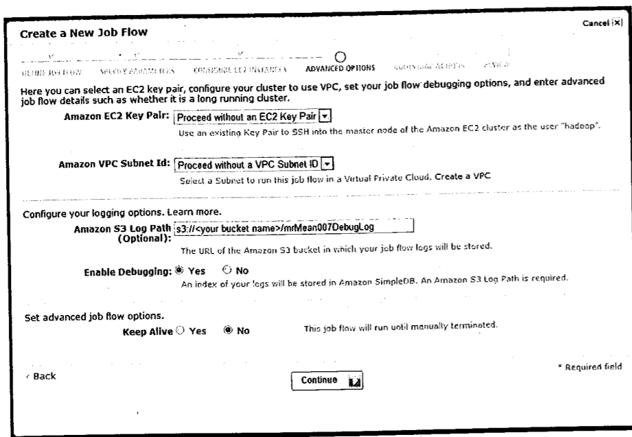
图15-7 EMR的高级选项页面，可以设定调试文件的存放位置，也可以设定继续自动运行机制。作业失败还可以设定登录服务器所需的登录密钥。如果想检查代码的运行环境，登录服务器再查看是个很好的办法
