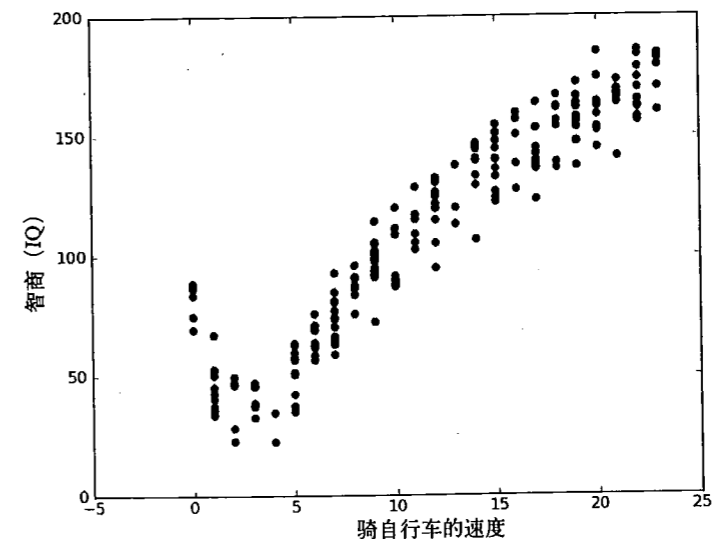
图9-6 人们骑自行车的速度和他们智商之间的关系数据。该数据用于比较树回归模型和普通的线性回归模型
