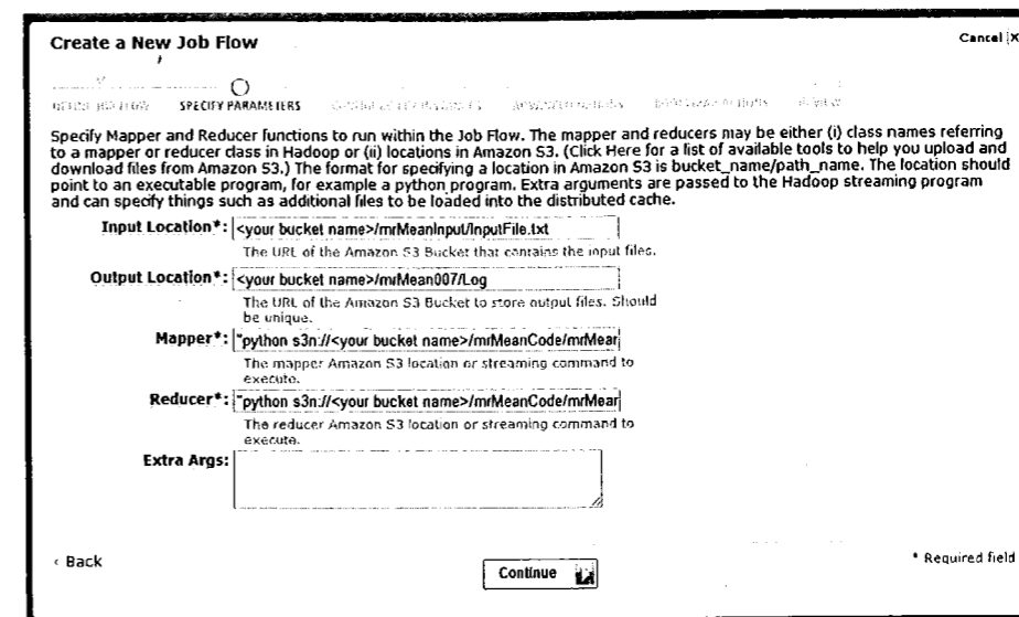
图15-5 EMR的指定参数页面
