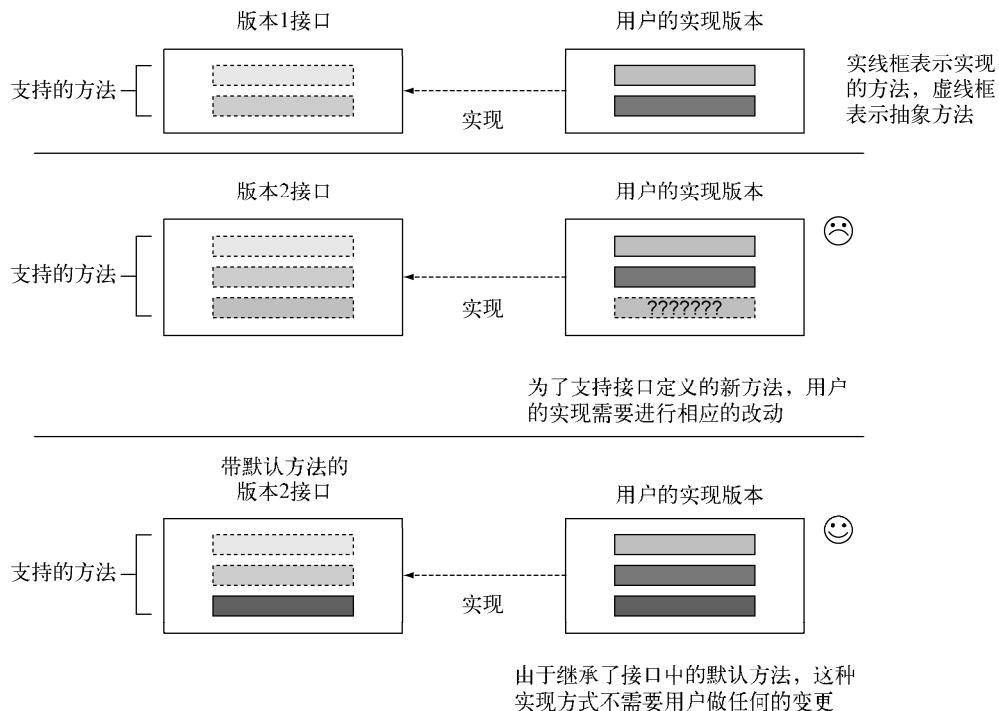
图9-1 向接口添加方法
